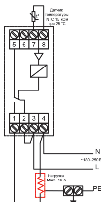
DEVIreg™ 330 (-10 ... 10 °C; 60 ... 160 °C)
